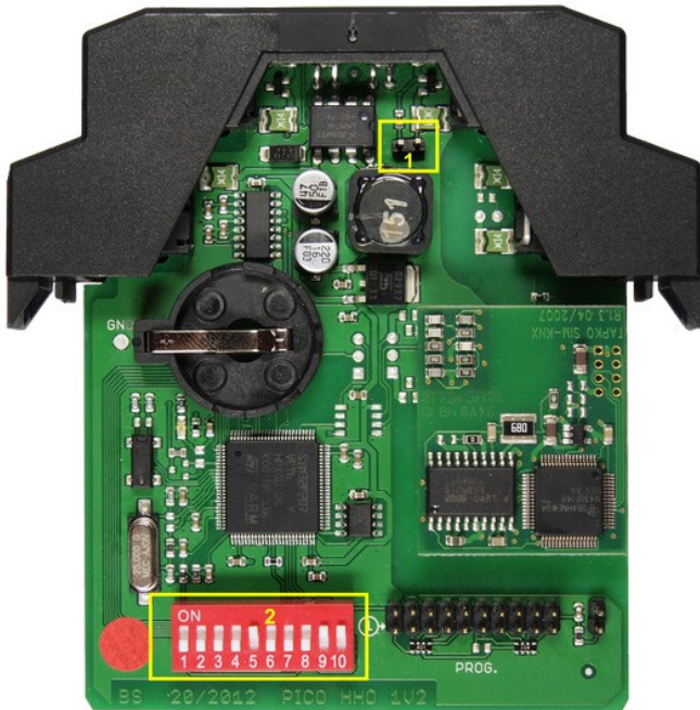
2 - Kodierschalter BACnet Parameter
